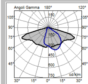
STU-M Optic
