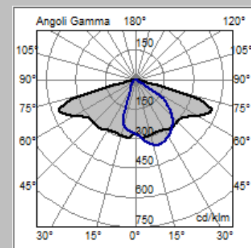
STU-M Optic
